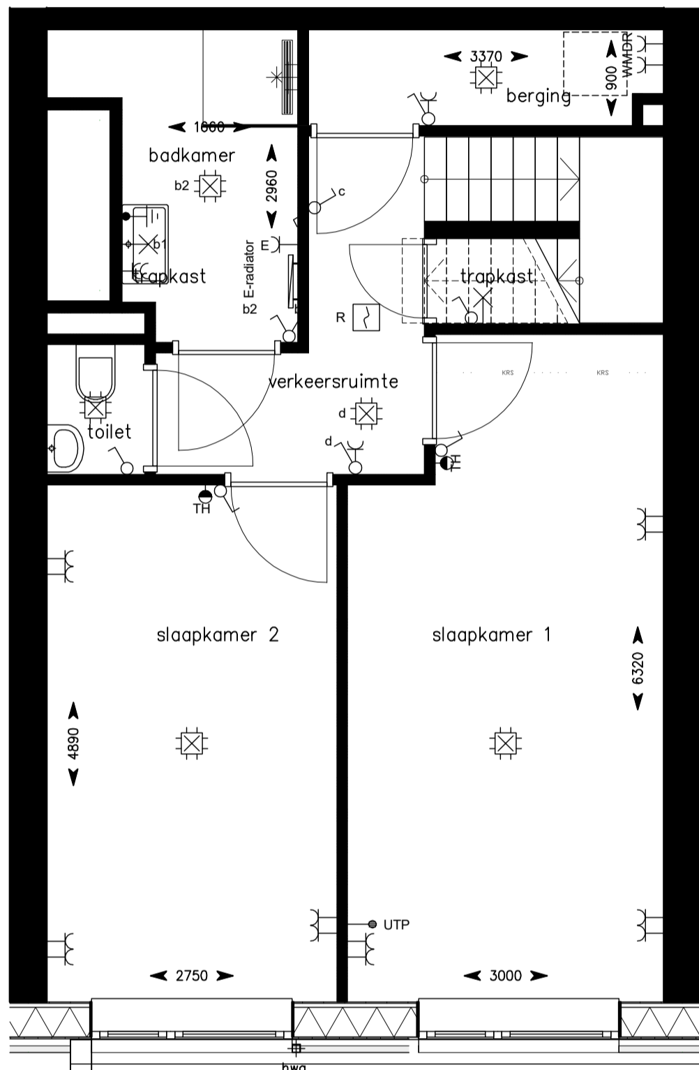
1e Verdieping
