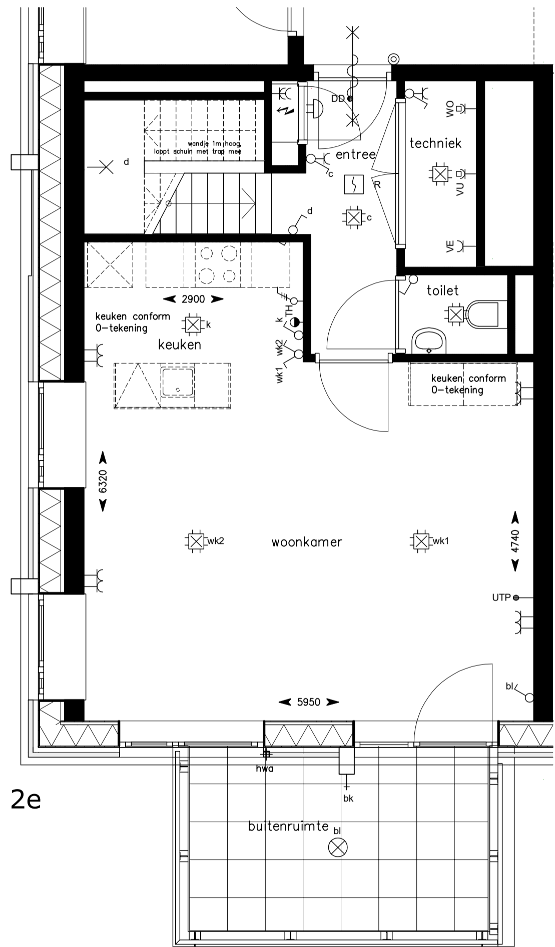
2e Verdieping
