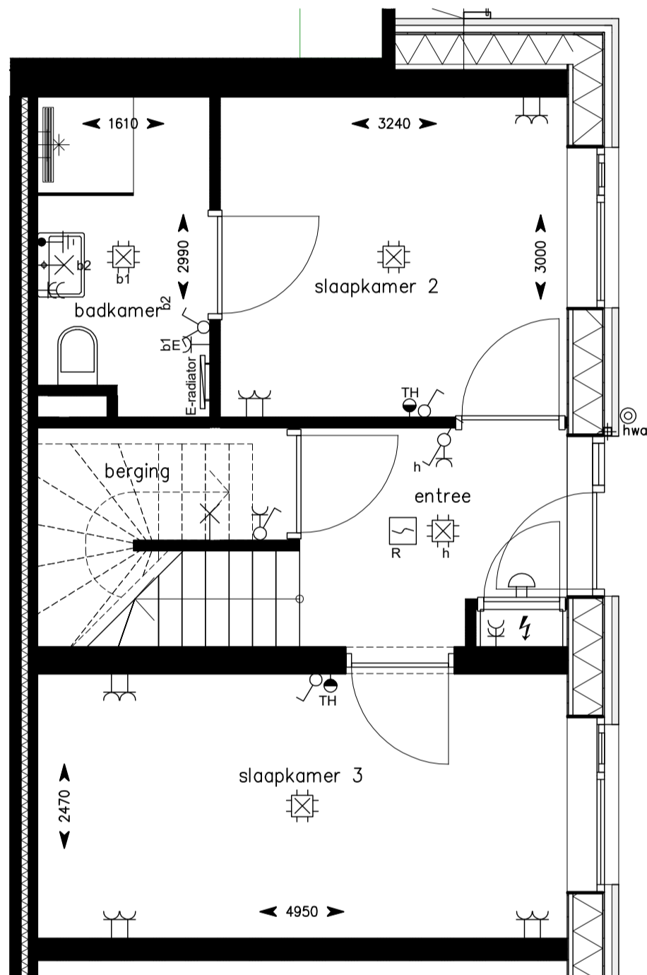
Begane grond
