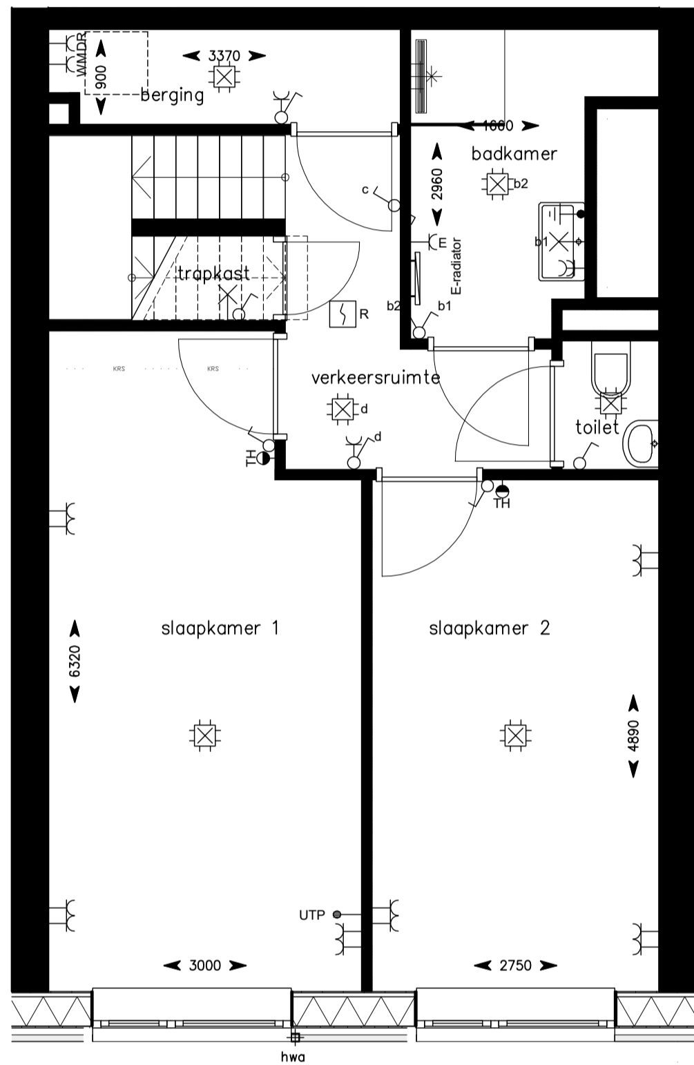
1e Verdieping
