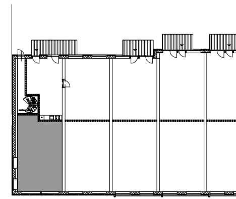
1e Verdieping
