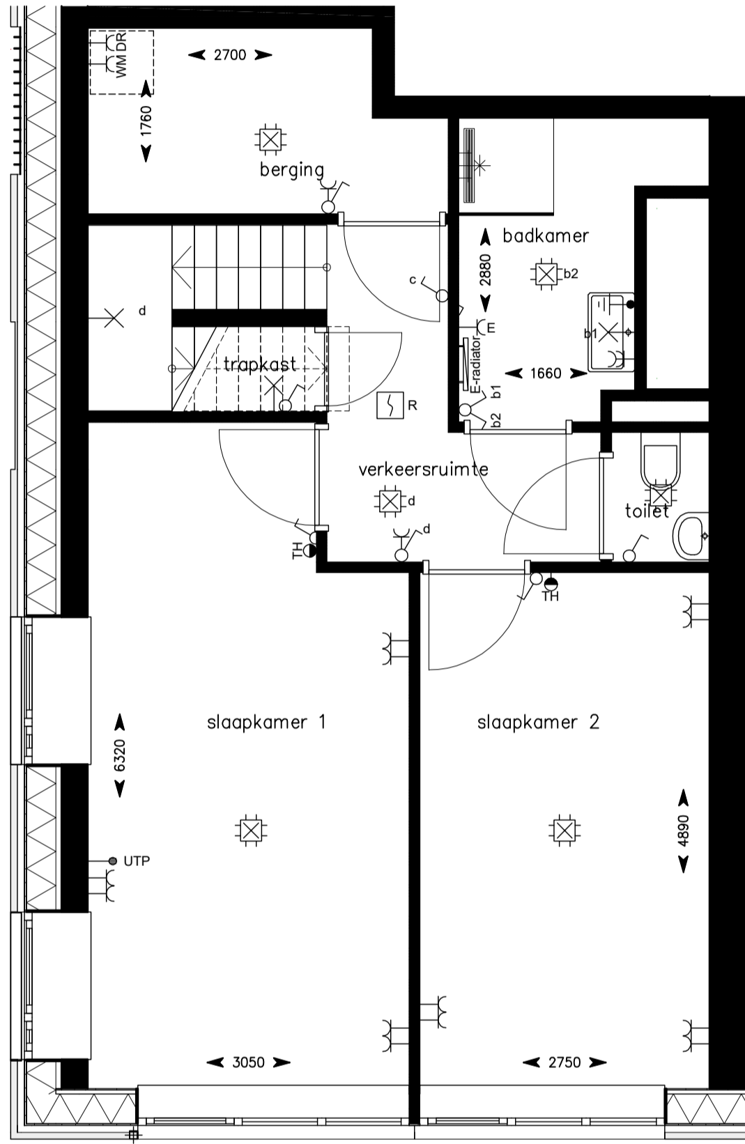
1e Verdieping
