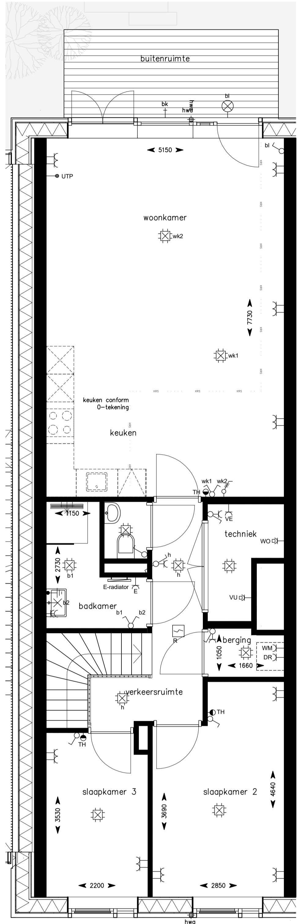
1e Verdieping
